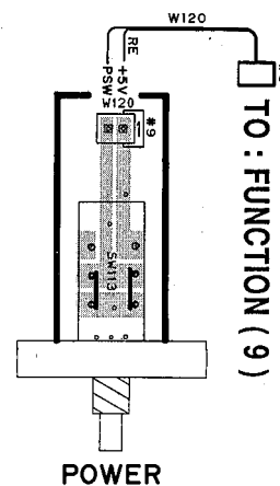
MAIN P. C. B. ( 7 )
