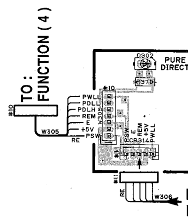
FUNCTION P. C. B. ( 8 )
